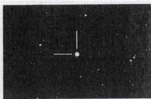
Champ de U Sco avant et après l'éruption
