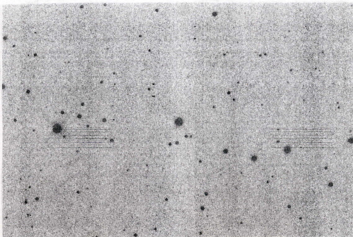
SS Cyg au maximum à JJ.55 399
