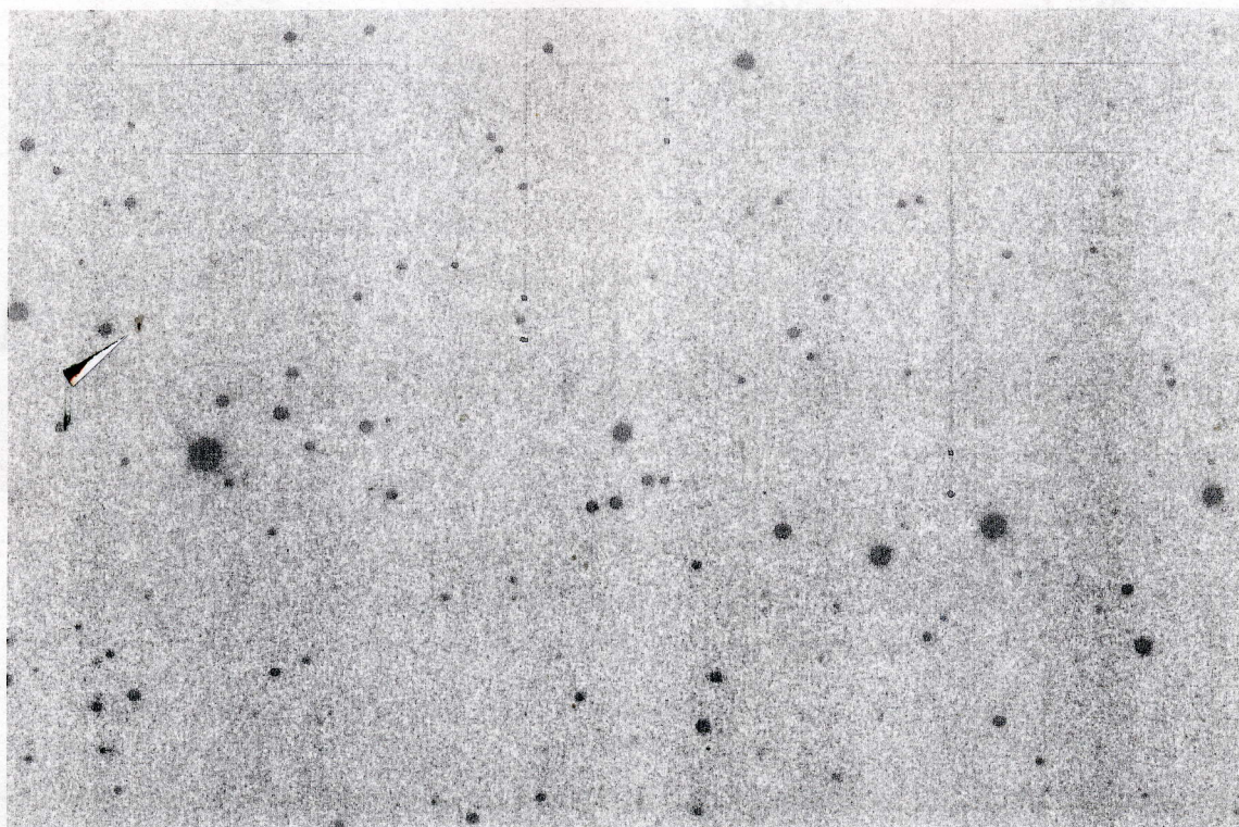
SS Cyg au minimum à JJ.55 396
