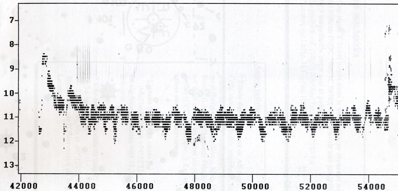
COURBE DE LUMIERE DE CI Cygni selon l'AFOEV (d'après Scw)
