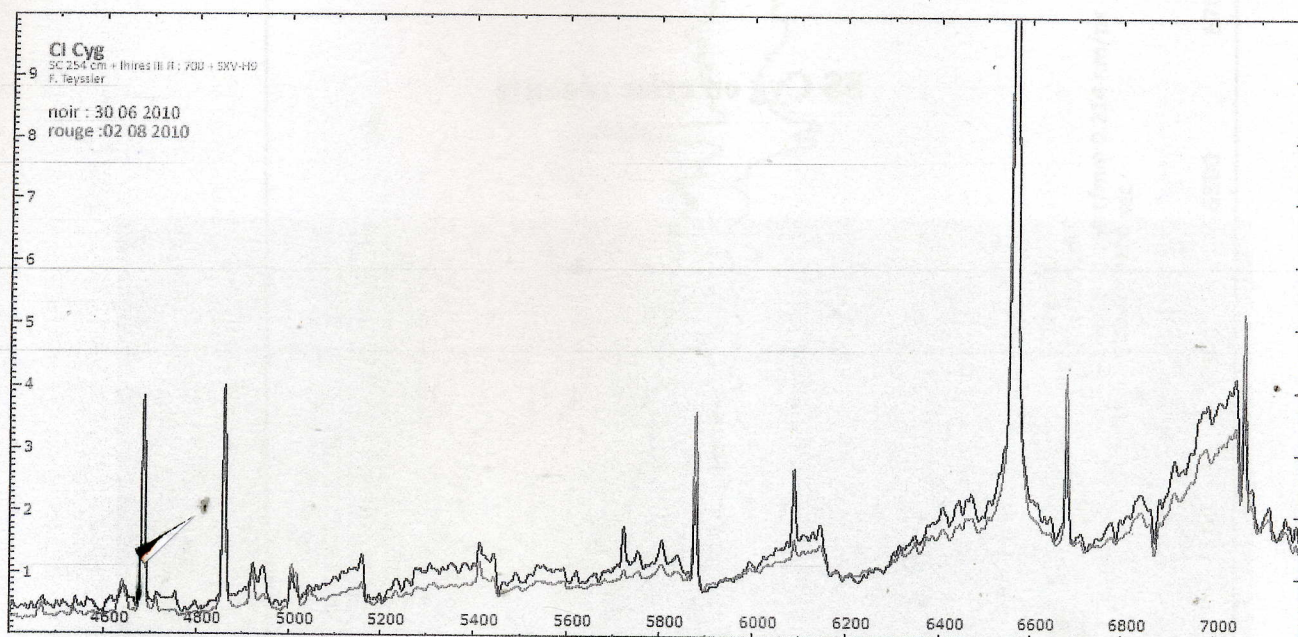
2 spectres de CI Cyg (F.Teyssier)
